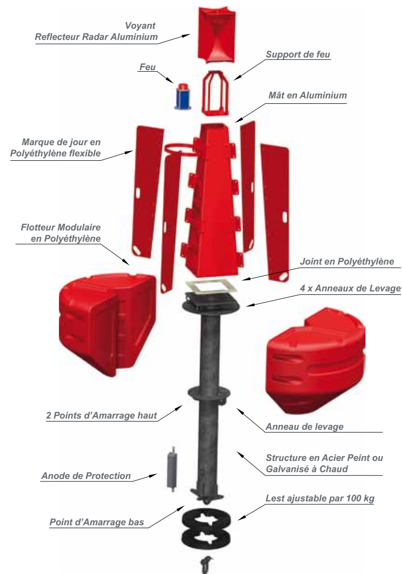
Vue éclatée d'une JET 2500 Q PF3 STD
