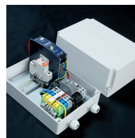
PS 120 Fuente de alimentación de 120 VA
